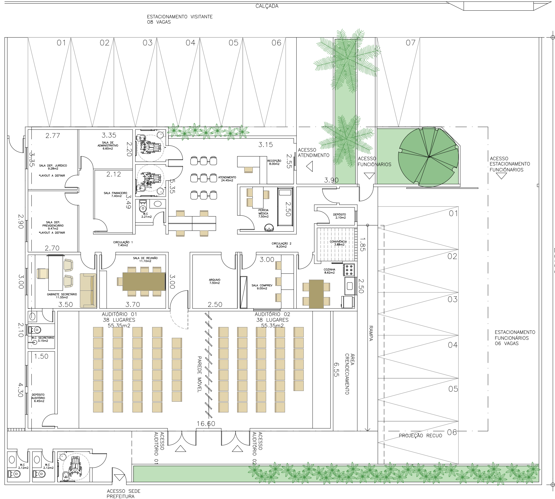
01 PLANTA BAIXA ESCALA 1/125
